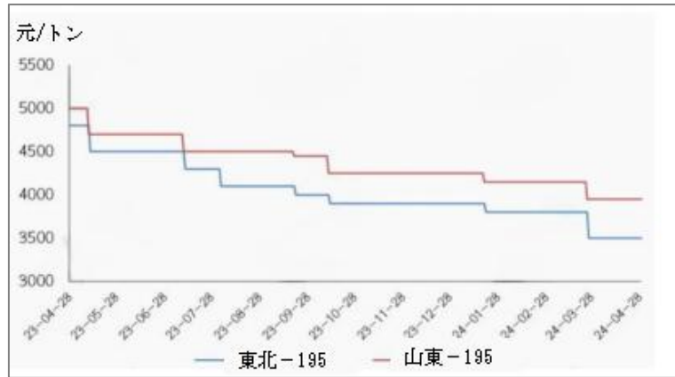
図2. 中国の鱗片状黒鉛の価格の推移 (2023年4月~2024年4月)
