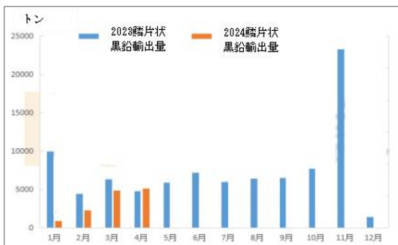
図1. 中国の鱗片状黒鉛の輸出量の推移（2023年1月~2024年4月）
