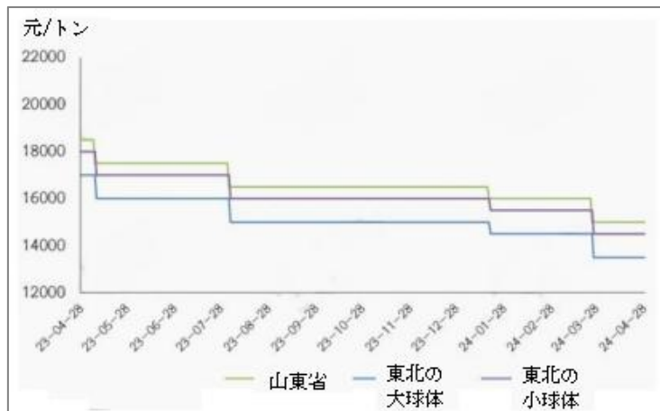
図2. 中国の鱗片状黒鉛の価格の推移 (2023年4月~2024年4月)
